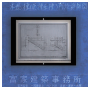
■矢田屋松濤園 階段詳細図 1966
